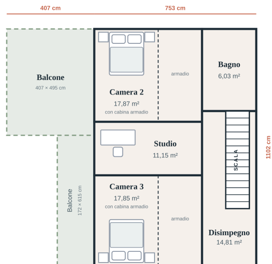
HUMAN-HABITAT - CASA A GIORNICO Pianta piano primo
